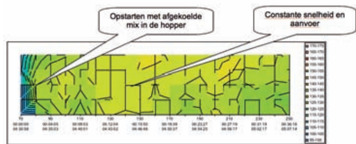
Figuur 3: Temperatuurcontourenkaart, woensdag strook 2
